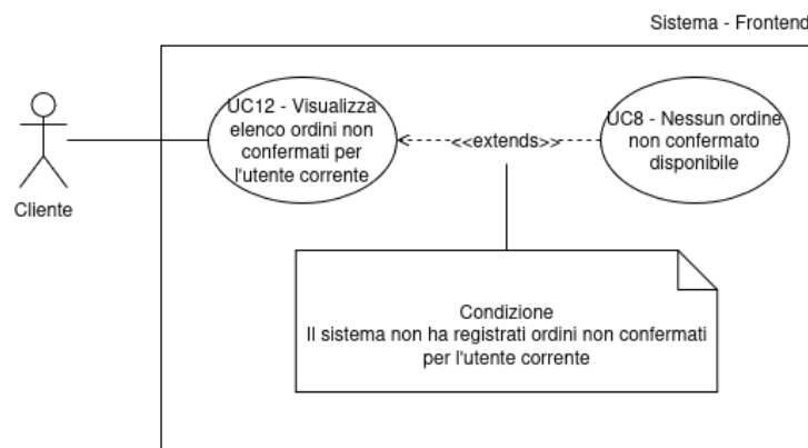
Figura 13: UC12 - Visualizza elenco ordini non confermati
