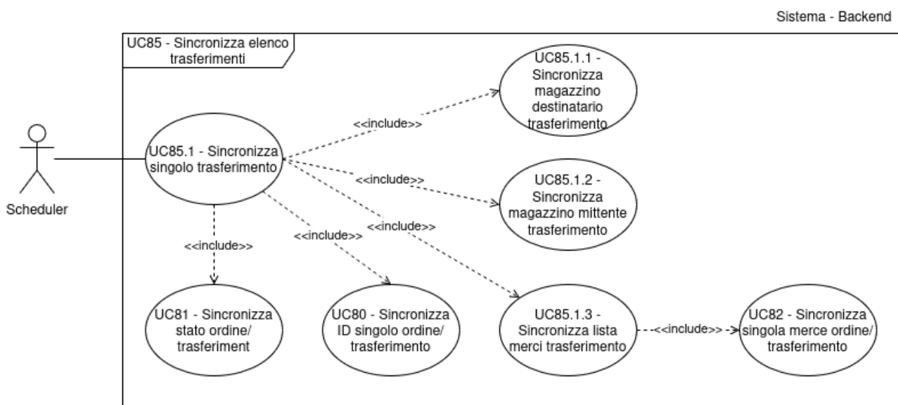
Figura 93: Inclusioni del Caso d'Uso n.85: UC85.1 e relative inclusioni
