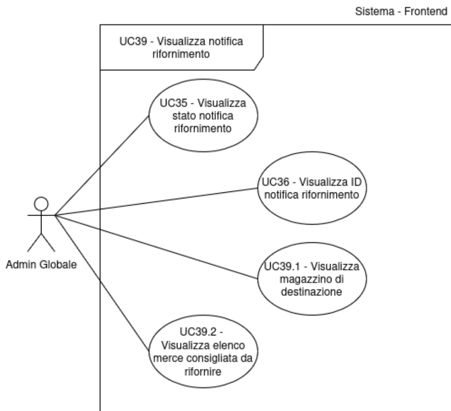
Figura 39: Inclusione del Caso d'Uso n.39: UC35, UC36, UC39.1 e UC39.2
