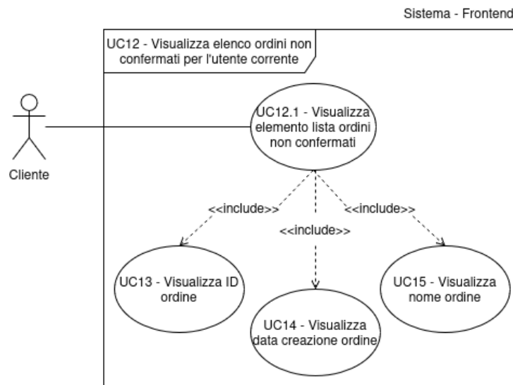
Figura 14: Inclusione del Caso d'Uso n.12: UC12.1
