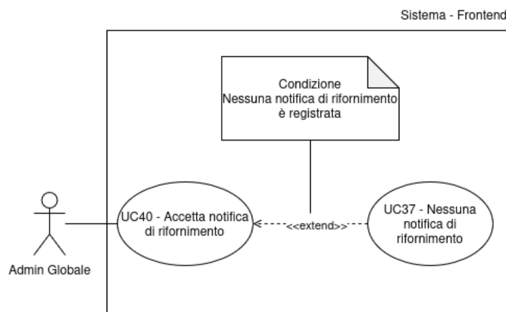
Figura 41: UC40 - Accetta notifica di rifornimento
