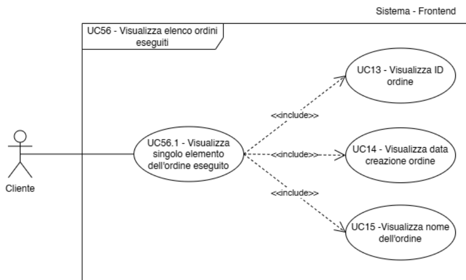
Figura 59: Inclusioni del Caso d'Uso n.56: UC56.1
