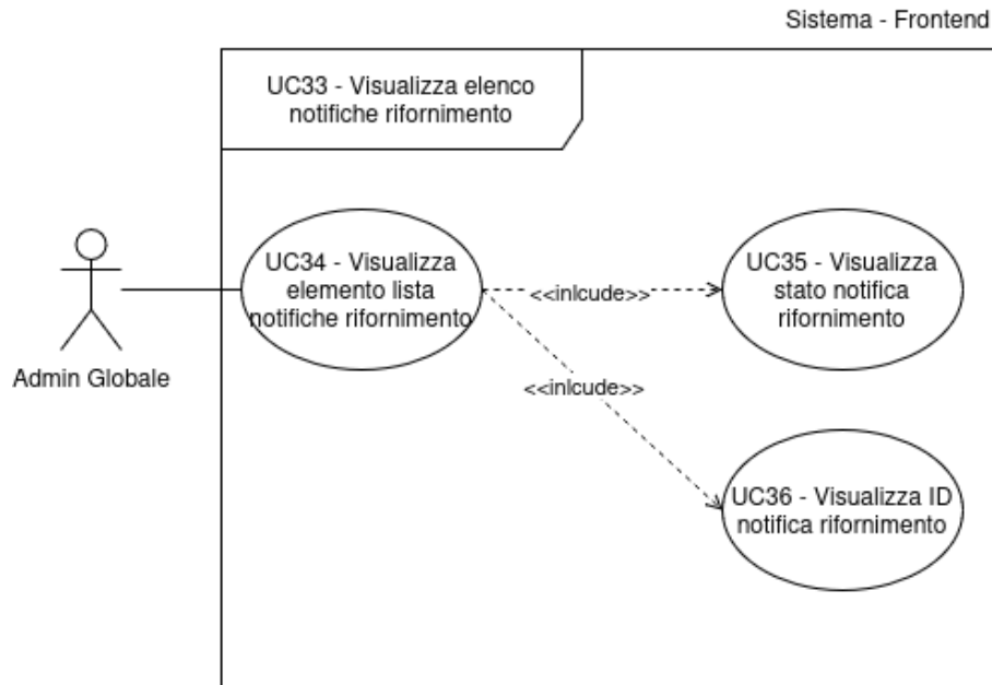
Figura 35: Inclusione del Caso d'Uso n. 33: UC34
