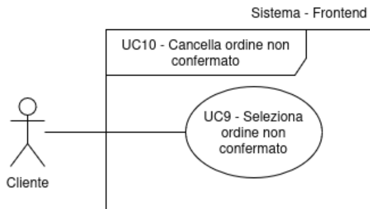
Figura 10: Inclusione del Caso d'Uso n.10: UC9
