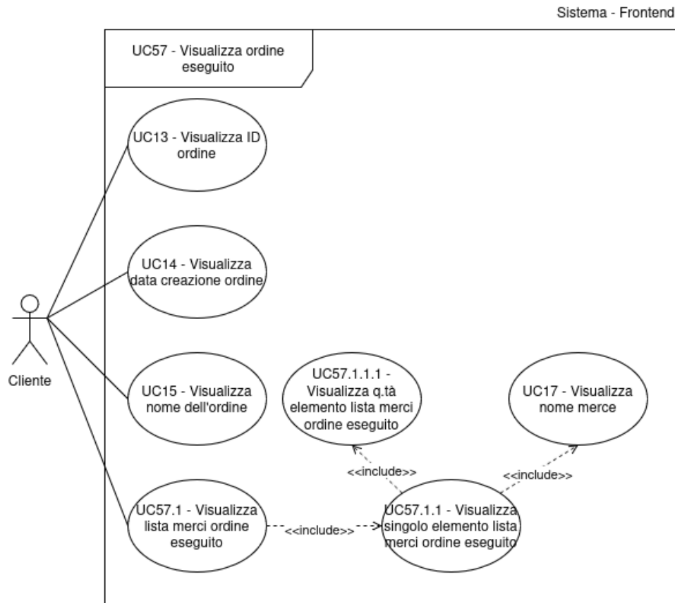
Figura 61: Inclusioni del Caso d'Uso n.57: UC13, UC14, UC15, UC57.1 e relative inclusioni
