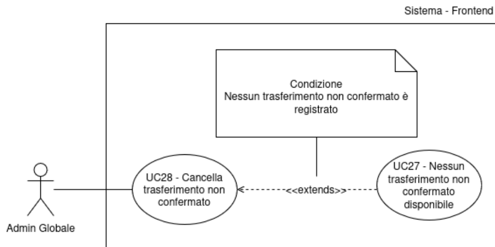
Figura 27: UC28 - Cancella trasferimento non confermato
