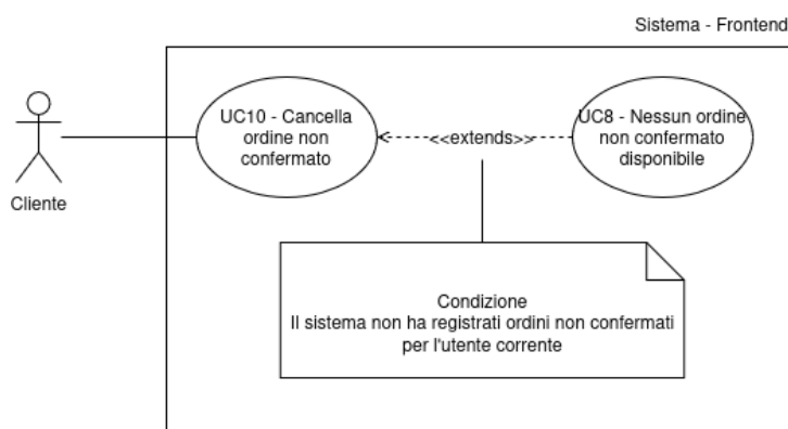
Figura 9: UC10 - Cancella ordine non confermato
