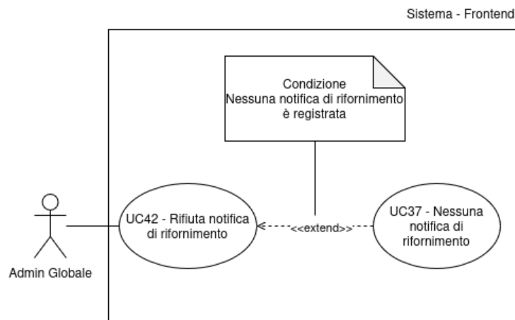
Figura 43: UC42 - Rifiuta notifica di rifornimento
