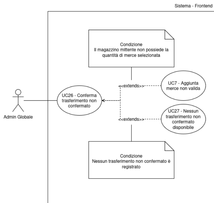
Figura 25: UC26 - Conferma trasferimento non confermato
