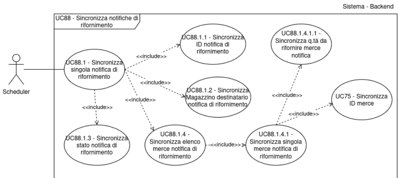
Figura 99: Inclusione nel Caso d'Uso n.88: UC88.1 e relative inclusioni
