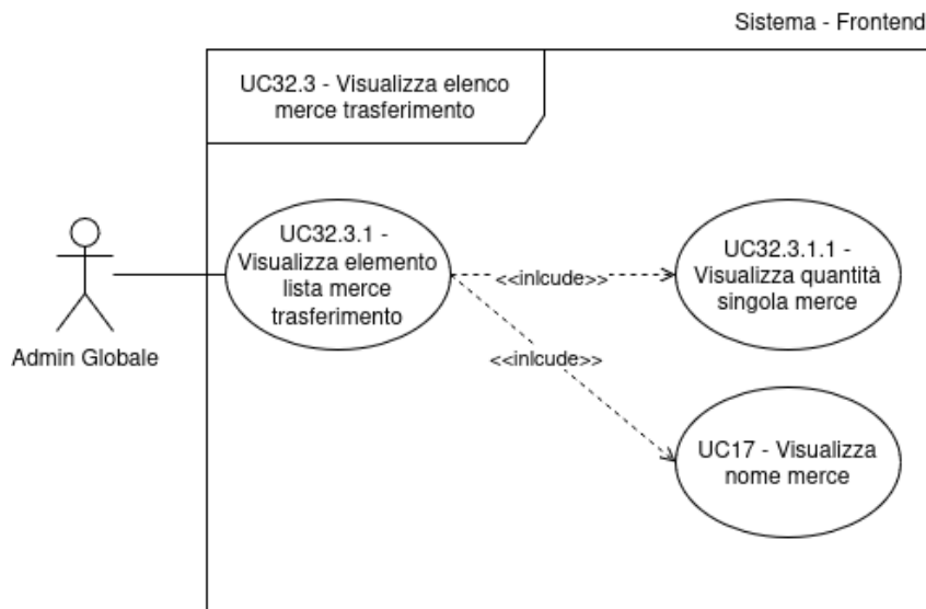
Figura 33: Inclusione del Caso d'Uso n.32.3: UC32.3.1 e relative inclusioni
