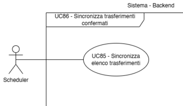
Figura 95: Inclusione nel Caso d'Uso n.86: UC85
