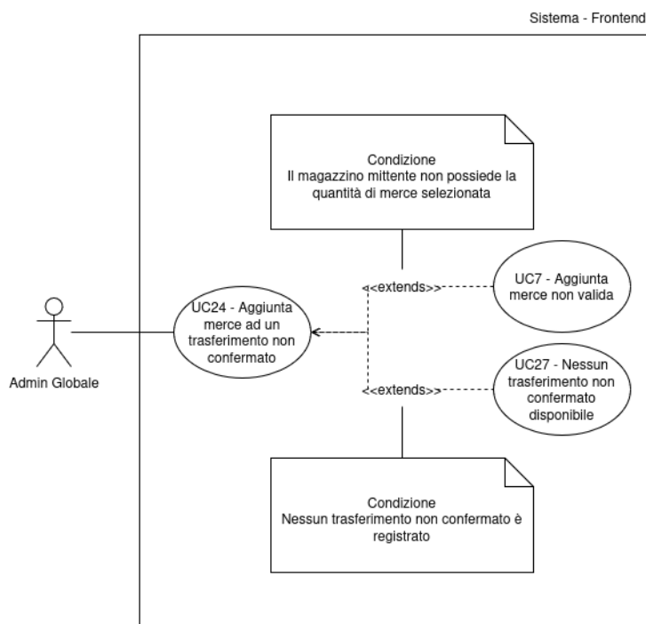
Figura 23: UC24 - Aggiunta merce ad un trasferimento non confermato
