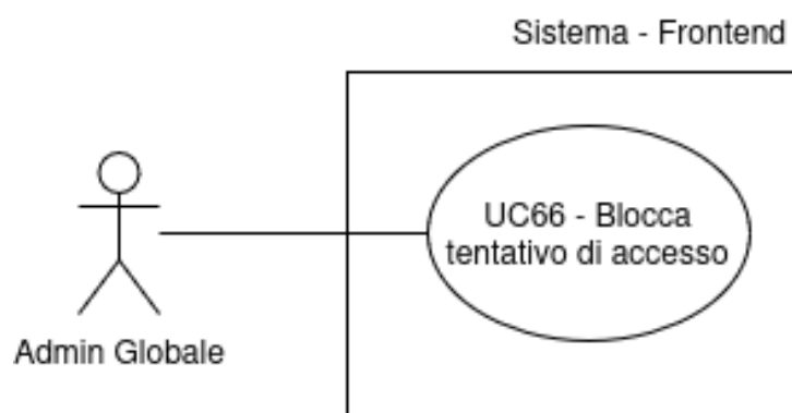
Figura 69: UC66 - Blocca tentativo di accesso
