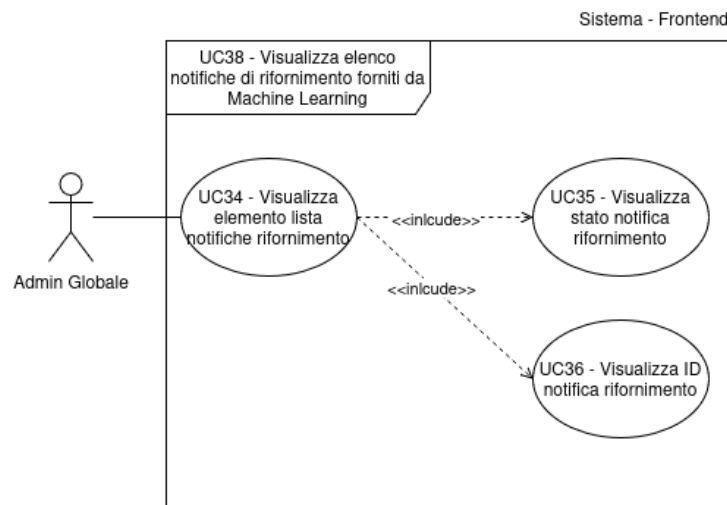
Figura 37: Inclusione del Caso d'Uso n.38: UC34
