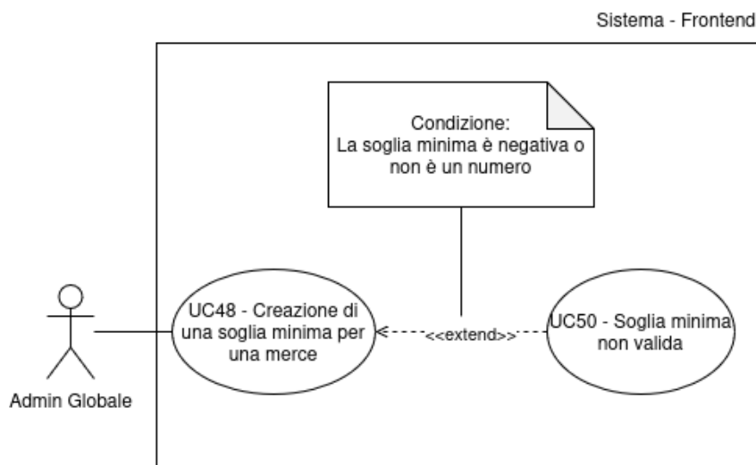
Figura 49: UC48 - Creazione di una soglia minima per una merce
