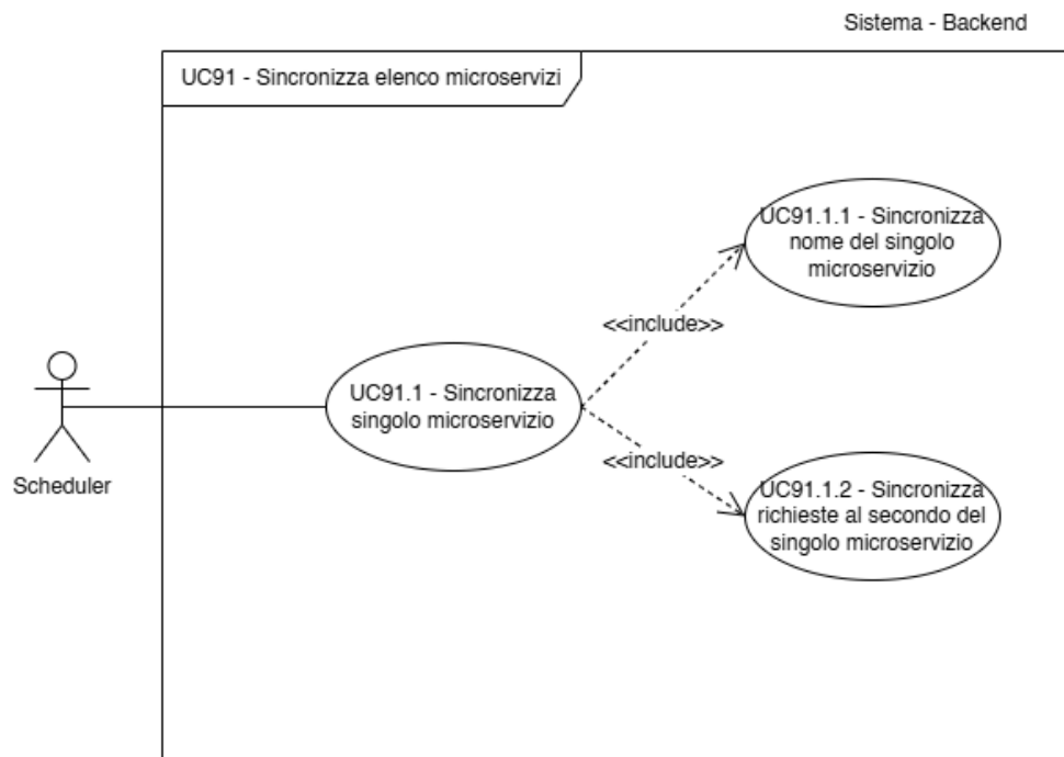
Figura 105: Inclusioni nel Caso d'Uso n.91: UC91.1 e relative inclusioni
