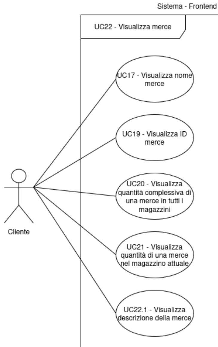
Figura 20: Inclusioni del Caso d'Uso n.22: UC17, UC19, UC20, UC21 e UC22.1
