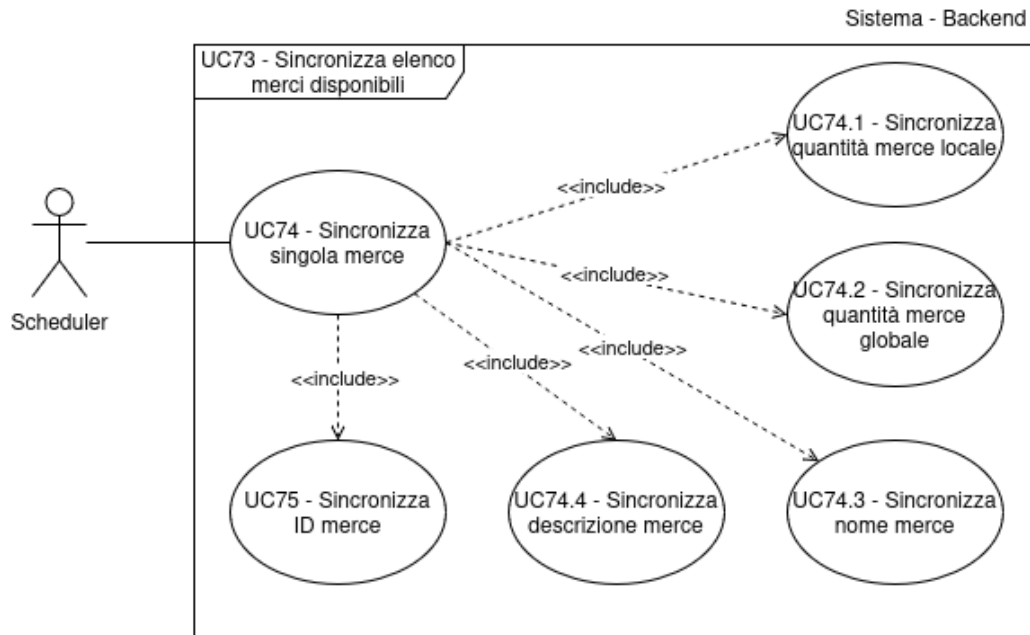
Figura 78: Inclusioni del Caso d'Uso n.73: UC74 e relative inclusioni
