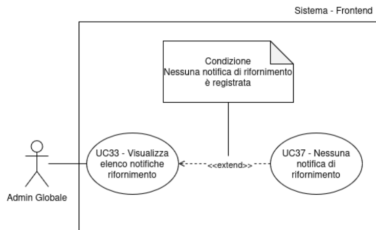
Figura 34: UC33 - Visualizza elenco notifiche rifornimento
