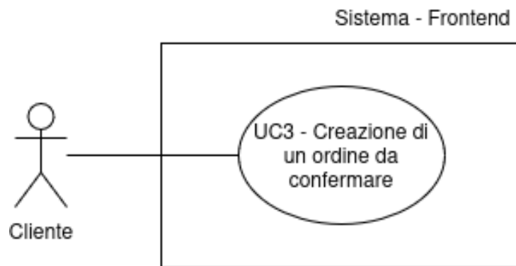
Figura 5: UC3 - Creazione di un ordine da confermare
