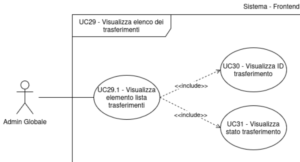
Figura 30: Inclusione del Caso d'Uso n. 29: UC29.1
