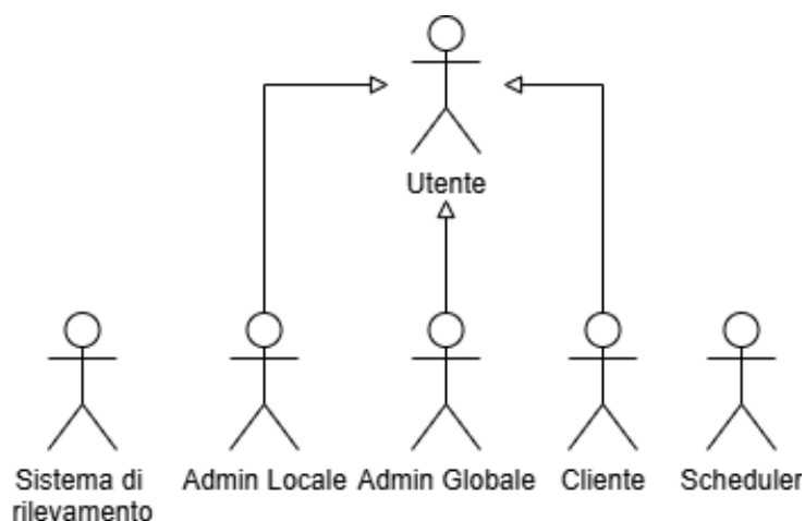
Figura 1: Diagramma degli attori principali
