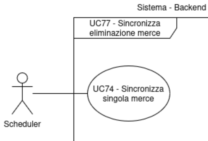
Figura 82: Inclusioni del Caso d'Uso n.77: UC74
