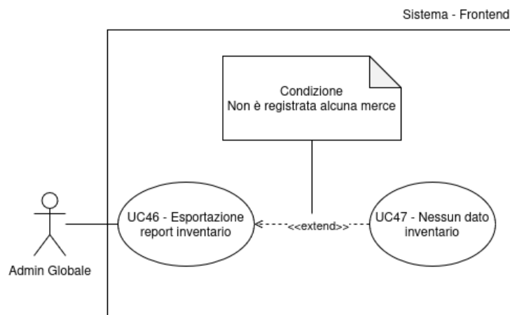
Figura 48: UC46 - Esportazione report inventario
