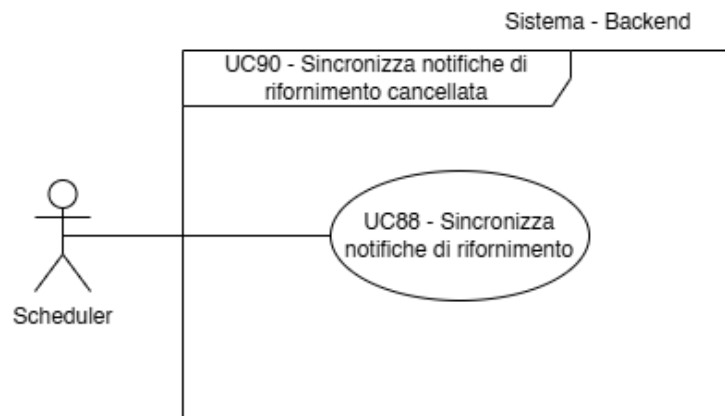
Figura 103: Inclusione nel Caso d'Uso n.90: UC88
