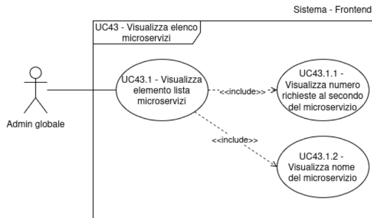
Figura 46: Inclusioni del Caso d'Uso n.43: UC43.1
