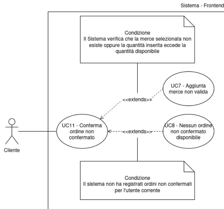
Figura 11: UC11 - Conferma ordine non confermato
