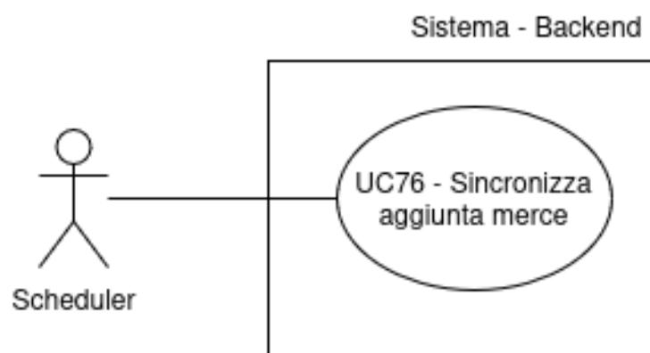
Figura 79: UC76 - Sincronizza aggiunta merce
