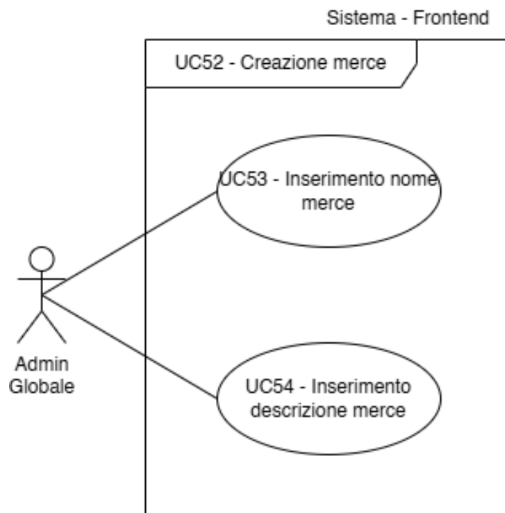
Figura 55: Inclusioni del Caso d'Uso n.52: UC53 e UC54
