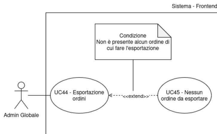
Figura 47: UC44 - Esportazione ordini
