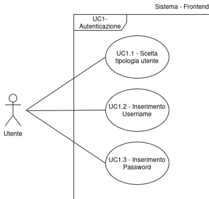
Figura 4: Inclusioni del Caso d'Uso n.1: UC1.1, UC1.2, UC1.3
