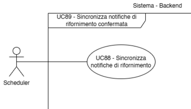
Figura 101: Inclusione nel Caso d'Uso n.89: UC88
