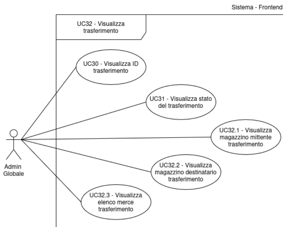
Figura 32: Inclusione del Caso d'Uso G n.32: UC30, UC31, UC32.1, UC32.2 e UC32.3
