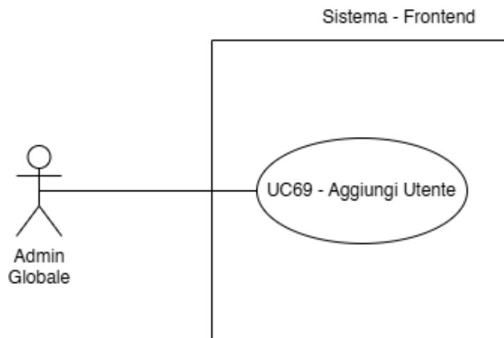
Figura 73: UC69 - Aggiungi nuovo utente
