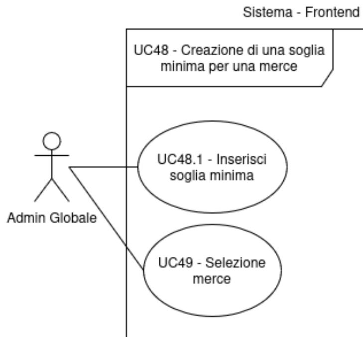
Figura 50: Inclusioni del Caso d'Uso n.48: UC48.1 e UC49
