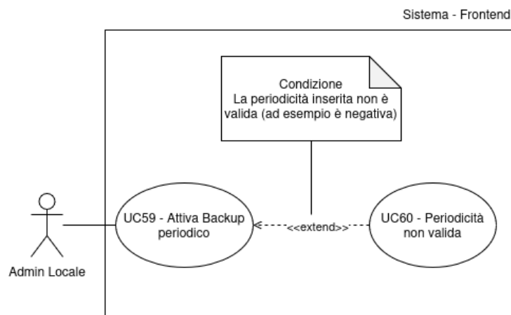
Figura 63: UC59 - Attiva Backup periodico
