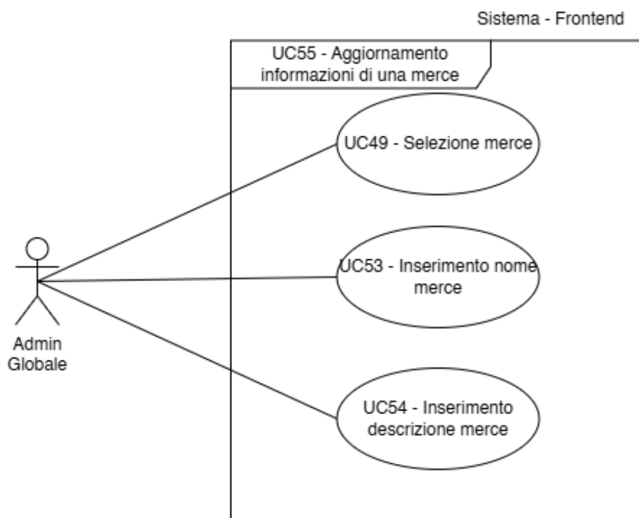
Figura 57: Inclusioni del Caso d'Uso n.55: UC49, UC53 e UC54
