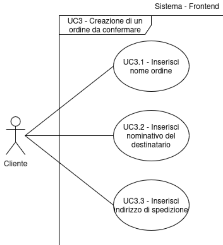
Figura 6: Inclusioni del Caso d'Uso n.3: UC3.1, UC3.2, UC3.3
