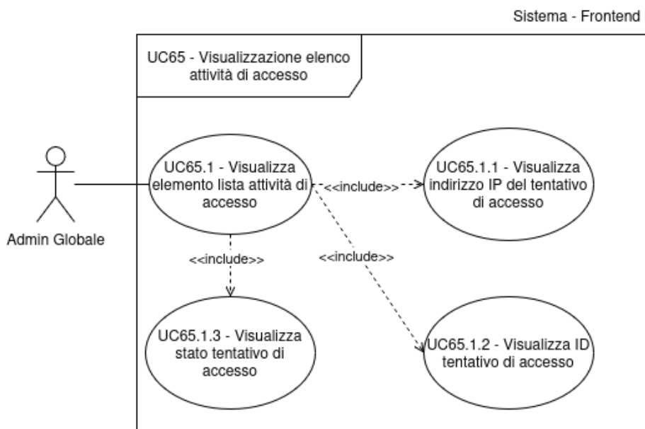
Figura 68: Inclusioni del Caso d'Uso n.65: 65.1 e relative inclusioni
