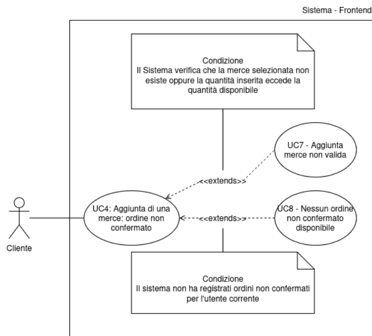
Figura 7: UC4 - Aggiunta di una merce ad un ordine non confermato
