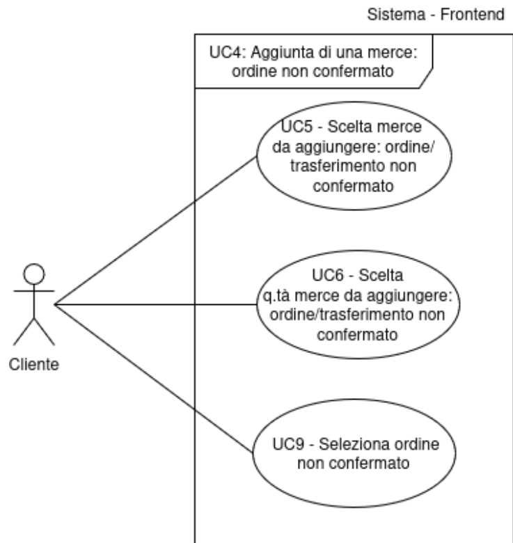
Figura 8: Inclusioni del Caso d'Uso n.4: UC5, UC6 e UC9
