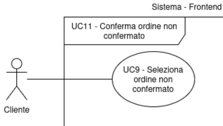
Figura 12: Inclusione del Caso d'Uso n.11: UC9
