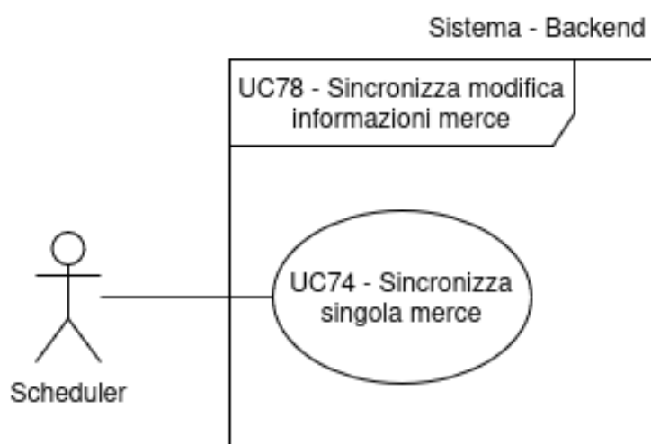
Figura 84: Inclusioni del Caso d'Uso n.78: UC74
