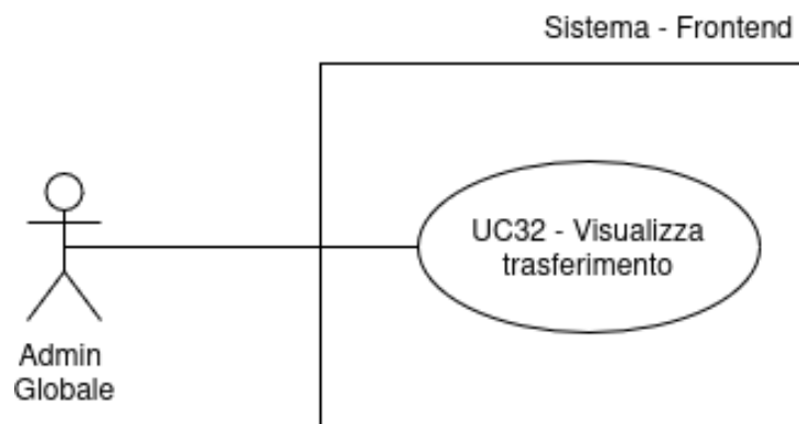
Figura 31: UC32 - Visualizza il singolo trasferimento
