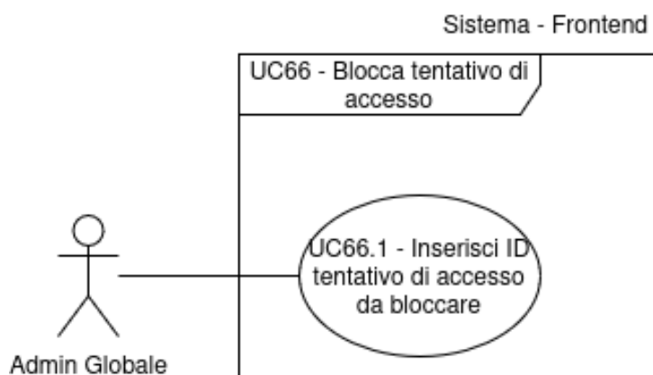
Figura 70: Inclusione del Caso d'Uso n.66: UC66.1
