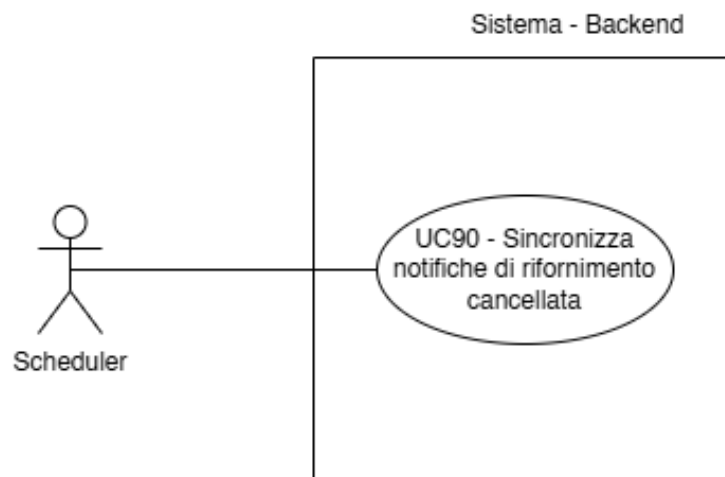
Figura 102: UC90 - Sincronizza notifiche di rifornimento cancellate
