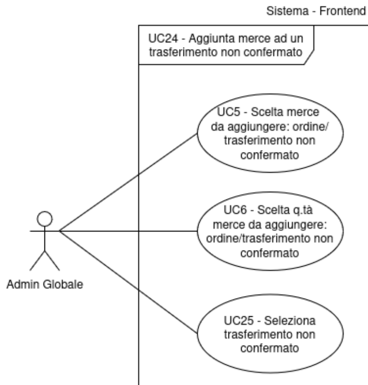
Figura 24: Inclusioni del Caso d'Uso n.24: UC5 , UC6 e UC25
