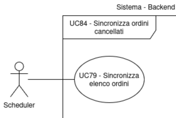
Figura 91: Inclusioni del Caso d'Uso n.84: UC79
