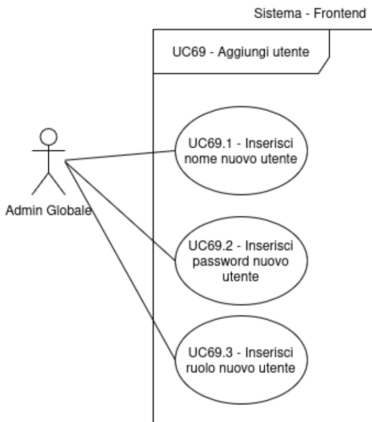
Figura 74: Inclusione del Caso d'Uso n.69: UC69.1, UC69.2, UC69.3
