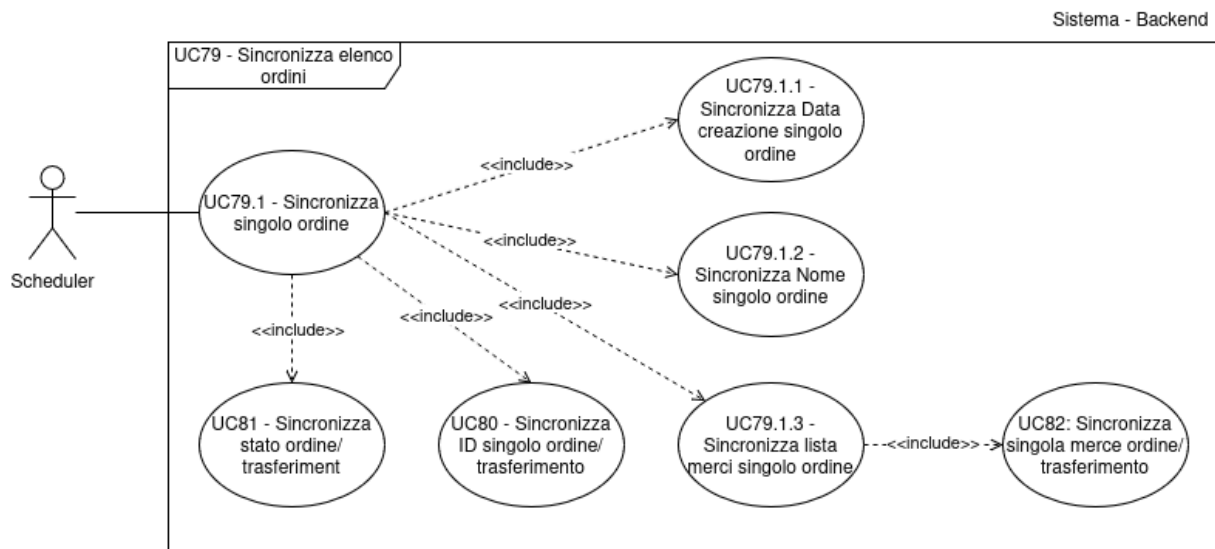
Figura 86: Inclusioni del Caso d'Uso n.79: UC79.1 e relative inclusioni
