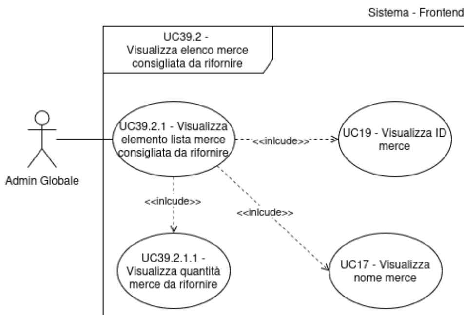
Figura 40: Inclusione del Caso d'Uso n.39.2: UC39.2.1
