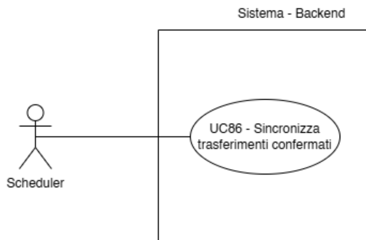
Figura 94: UC86 - Sincronizza trasferimenti confermati
