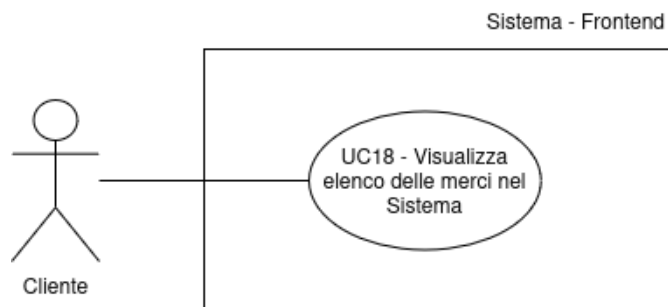
Figura 17: UC18 - Visualizza lista delle merci
