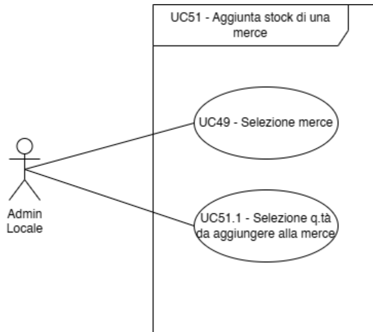
Figura 53: Inclusioni del Caso d'Uso n.51: UC49 e UC51.1
