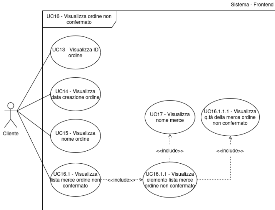
Figura 16: Inclusione del Caso d'Uso n.16: UC13, UC14, UC15, UC16.1
