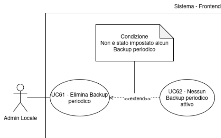
Figura 65: UC61 - Elimina Backup periodico
