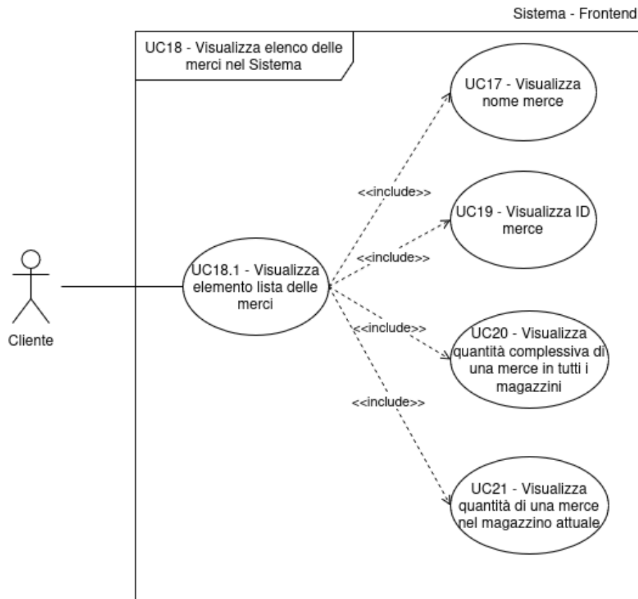
Figura 18: Inclusione del Caso d'Uso n.18: UC18.1
