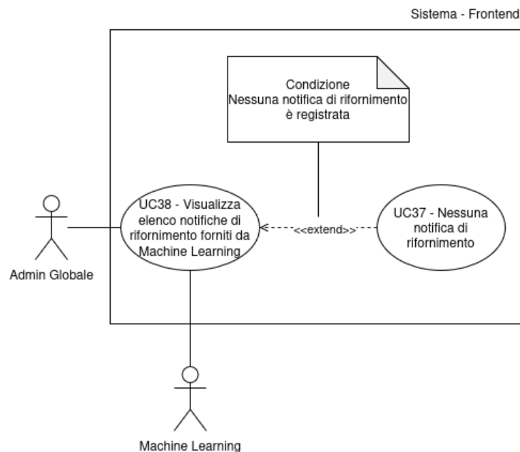
Figura 36: UC38 - Visualizza elenco notifiche di rifornimento con Machine Learning
