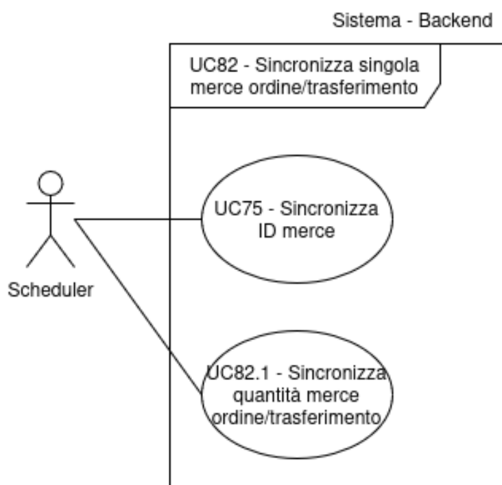
Figura 87: Inclusioni del Caso d'Uso n.82: UC75 e UC82.1
